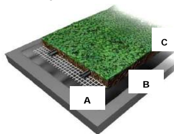
Figure 4 – Complexe de végétalisation Vertige®
